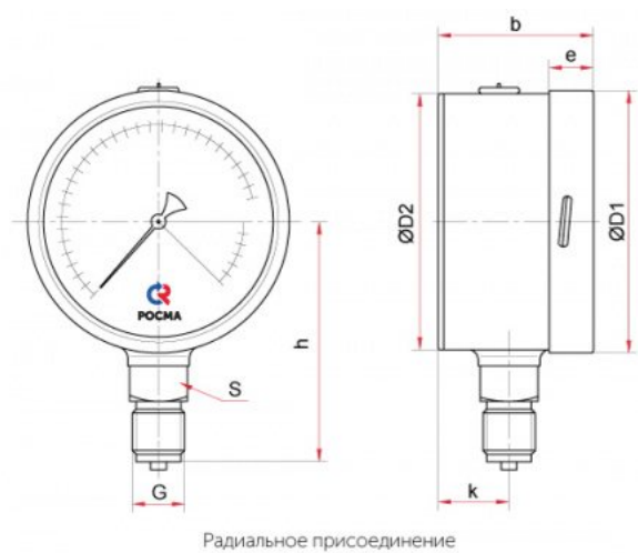
Основные размеры (мм), вес (кг), объём (мл)
